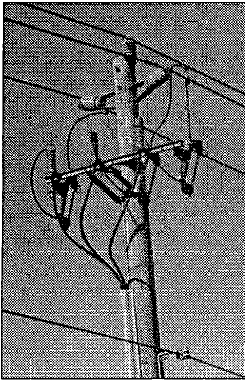
Riser pole
